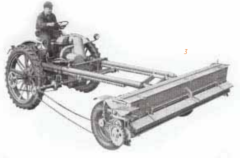
3 Frontanbau-Düngerstreuer BM 2 E, mit Geräteträger, 1956
